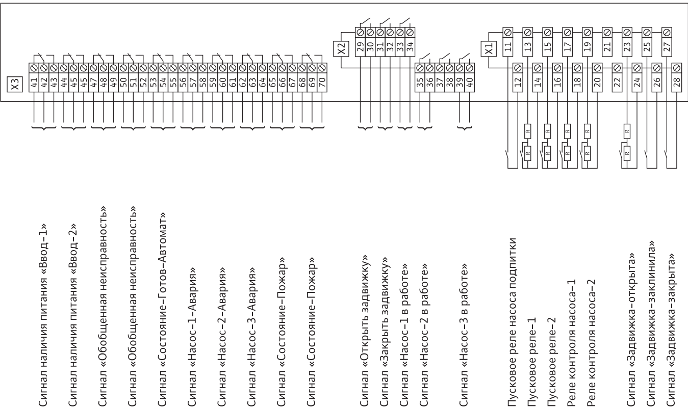
Схема подключения сигнальных цепей
