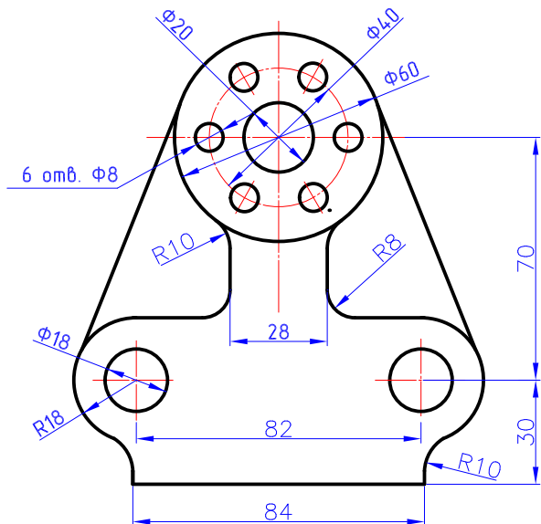
Стойка
