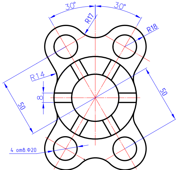
Крышка
