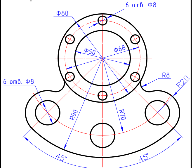
Корпус
