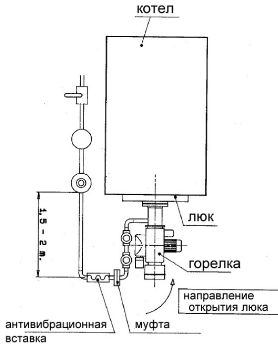
ВИД СБОКУ
