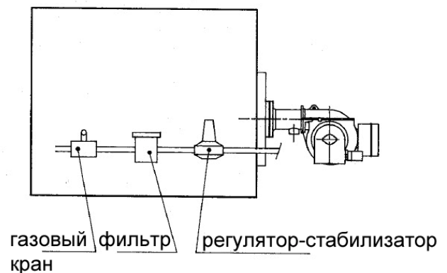
ВИД СБОКУ
