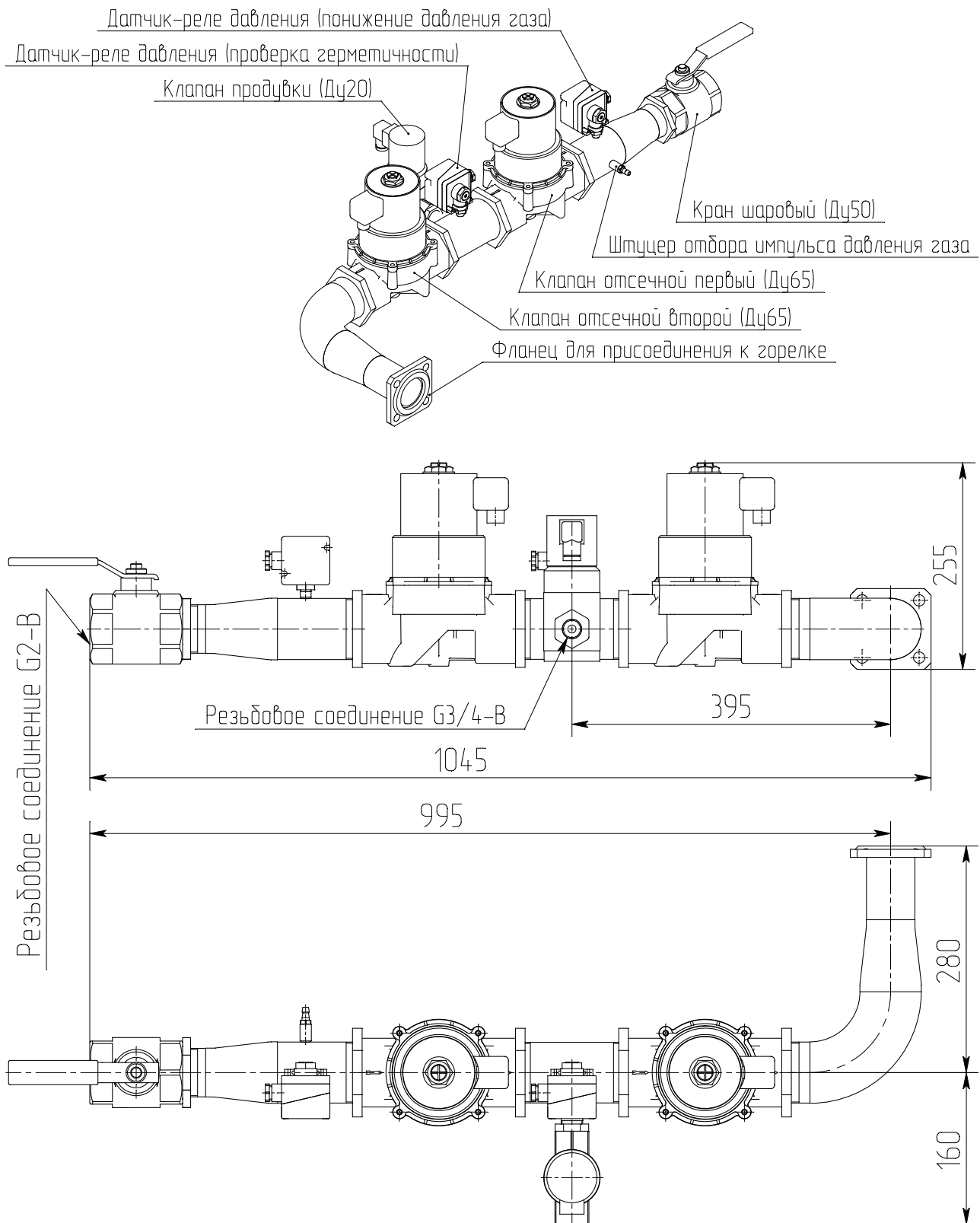
Рисунок В.3. Группа арматурная Са6.617.065 (Са6.617.065-02)
