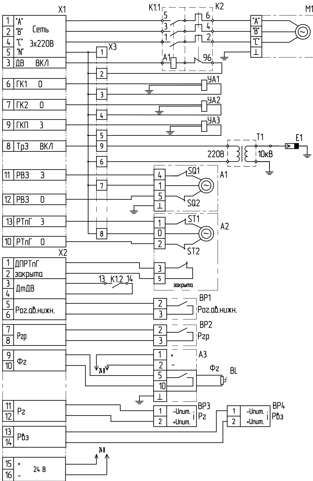
Схема электрическая принципиальная горелки ГБЛ
