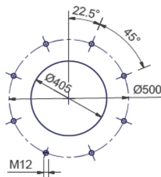
Рекомендуемая амбразура котла
