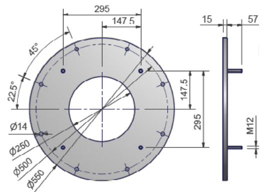
Рекомендуемый фланец горелки
