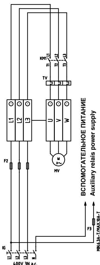
Рис. 12: Подключение электродвигателя
