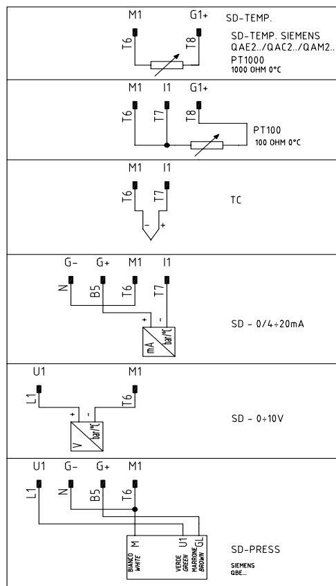
Рис. 18 - : Соединение датчиков
