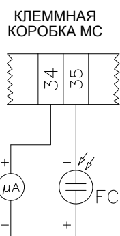
Рис. 31 - Контроль пламени с помощью фотозлемента QRA.
