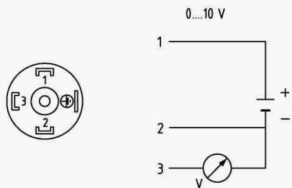
L-разъем DIN EN 175301-803
