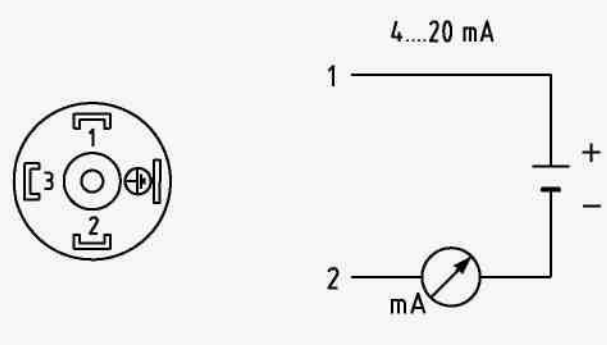
L-разъем DIN EN 175301-803
