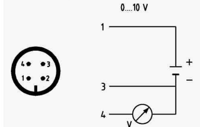
Разъем 4-pin M12 x 1
