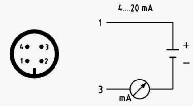
Разъем 4-pin M12 x 1
