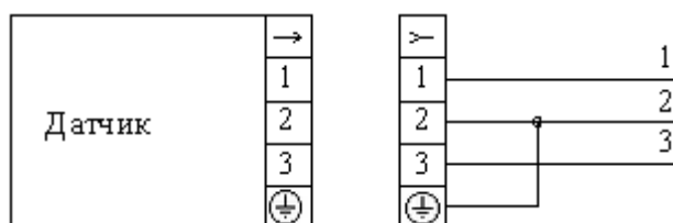
Рисунок В.3 Схема внешних электрических соединений для датчиков с протоколом обмена Mida/ UART с передачей информации об измеренном давлении по запросу
