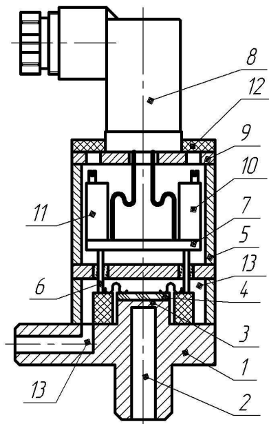
Рисунок 3- Датчик разности давлений МИДА-ДД-15
