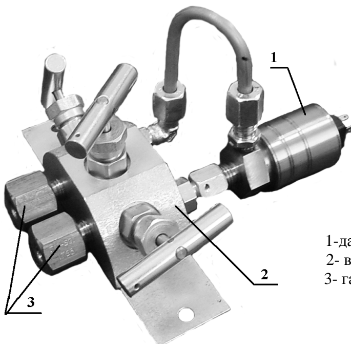
Рисунок Е.3 - Датчик МИДА-ДД-15 установленный на вентильный блок с двумя гасителями пульсаций
