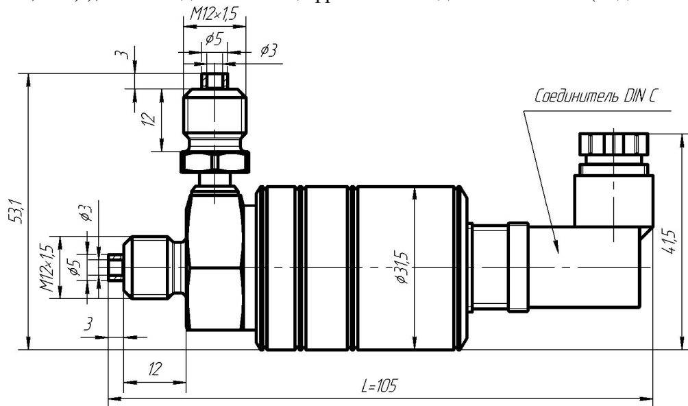
Рисунок Д.3 – Габаритные и присоединительные размеры датчиков МИДА-ДА-15, МИДА-ДА-15-Ех, МИДА-ДИ-15, МИДА-ДИ-15-Ех с выходным сигналом в виде напряжения постоянного тока и наличием пропорциональной зависимости от напряжения питания (код сигнала 055, 057), а также датчиков с цифровым выходным сигналом (код сигнала 061-064)
