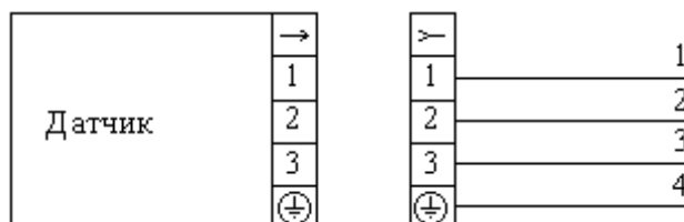
Рисунок В.1 Схема внешних электрических соединений для датчиков с выходным сигналом в виде напряжения постоянного тока
