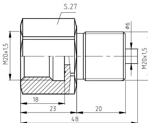
Рисунок Е.2- Габаритный чертеж гасителя пульсаций МИДА-ГП-501
