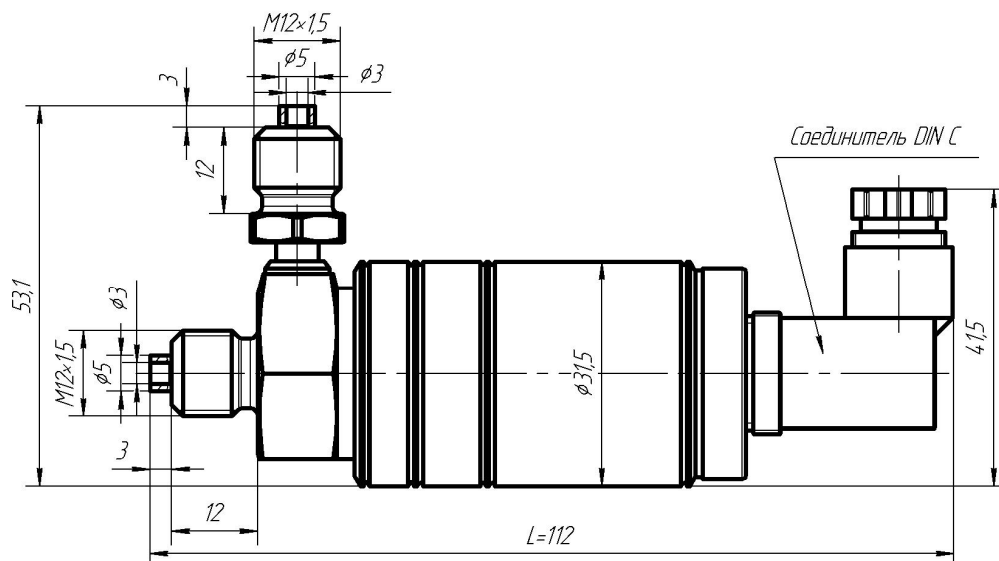
Рисунок Д.2 – Габаритные размеры датчика МИДА-ДД-15, МИДА-ДД-15-Ех с выходным сигналом в виде напряжения постоянного тока и наличием подстройки «нуля» и «диапазона» (код сигнала 051, 052)
