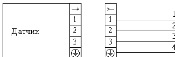
Рисунок В.2 Назначение контактов соединителя для датчиков с протоколом обмена Modbus/RS485 с передачей информации об измеренном давлении по запросу
