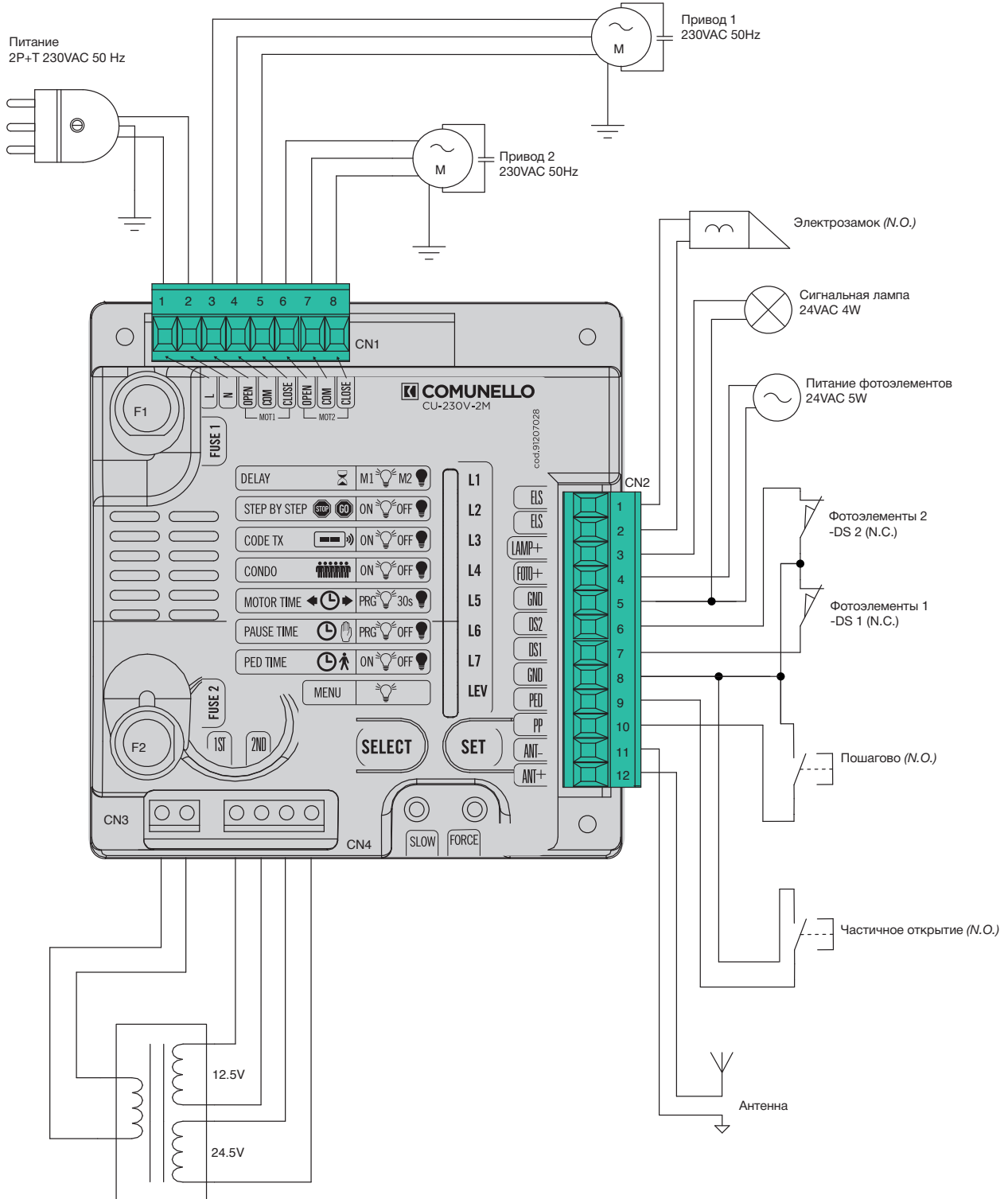
Трансформатор 230/24.5V - 0.4A; 12.5V - 0.17A
