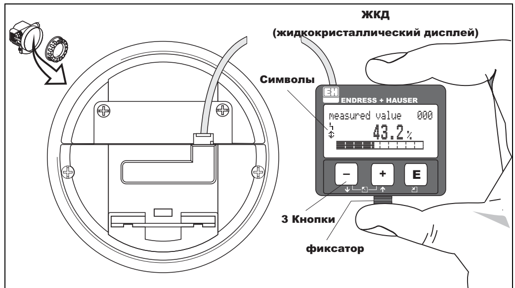
Рис. 1: Структура дисплея и органов управления
