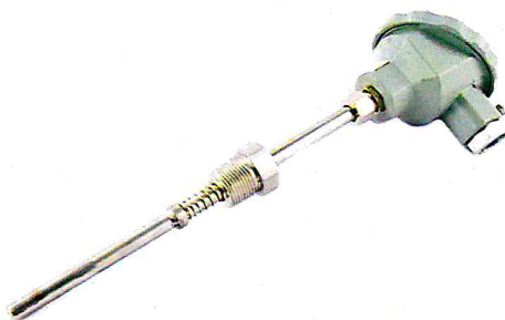
Рисунок 2 - Общий вид ТП модели ТП2
